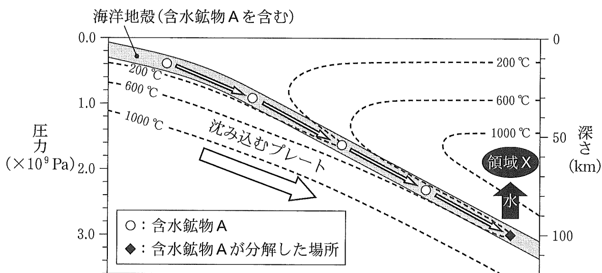
図2 ある沈み込み帯における断面図
