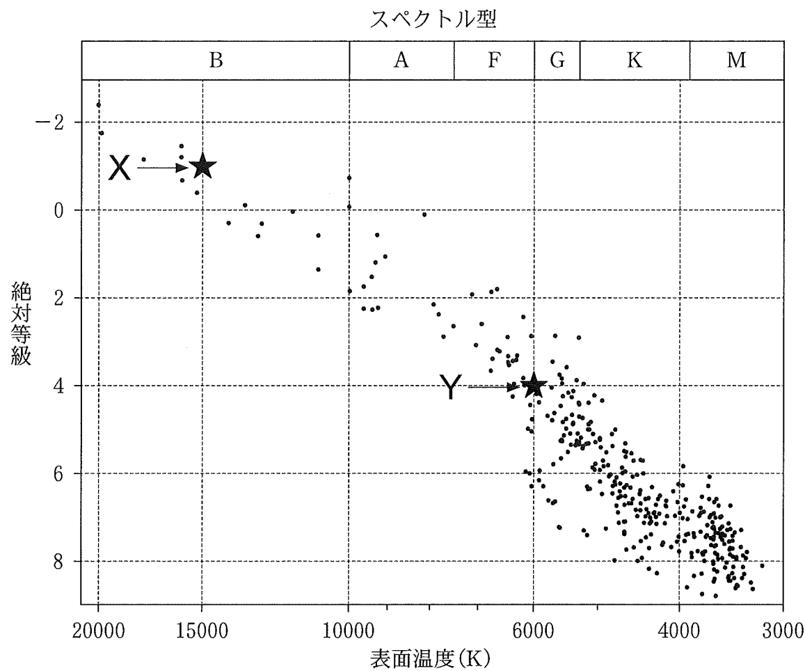
図 3 星団の HR 図
