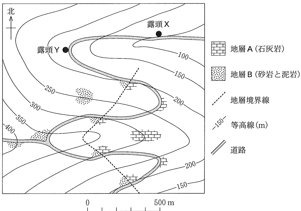
図3 ある地域の地形図と地層の分布
