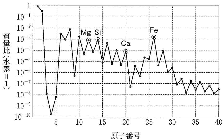
図 2 太陽大気の種類組成(水素に対する元素の質量比を示す)
