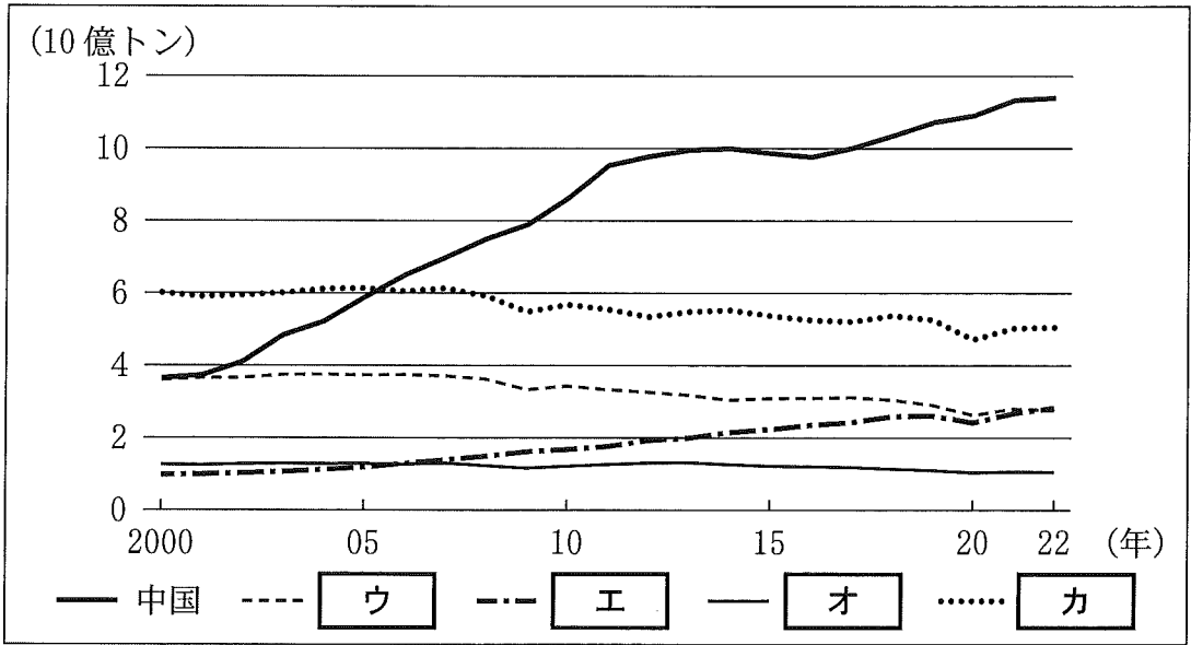
図2-1 二酸化炭素の総排出量
